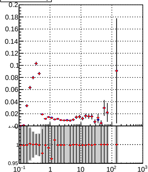
■ DQM_TT_mkFit-DQM_init_orig ■ DQM_TT_mkFit-DQM_init_mod
