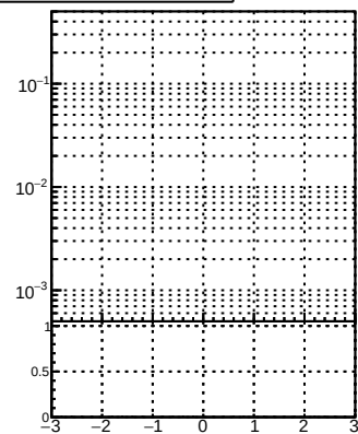
pT eta
