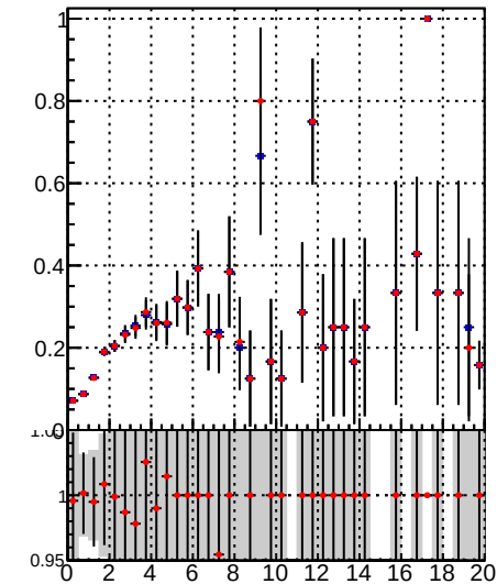
Fake rate vs. —●— DQM TT mkFit-DQM_init_orig —●— DQM TT mkFit-DQM_init_mod
