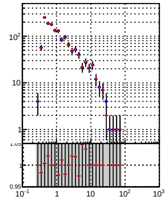
—•— DQM TT mkFit-DQM_init_orig —•— DQM TT mkFit-DQM_init_mod
