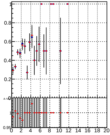
Fake rate vs. \bullet DQM TT mkFit-DQM_init_orig \bullet DQM TT mkFit-DQM_init_mod
