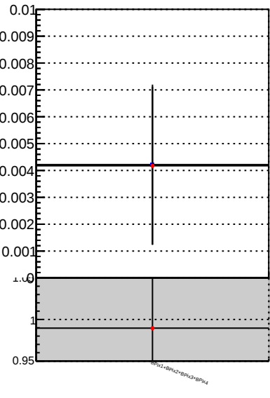
Fake rate vs. \bullet DQM TT mkFit-DQM_init_orig \bullet DQM TT mkFit-DQM_init_mod
