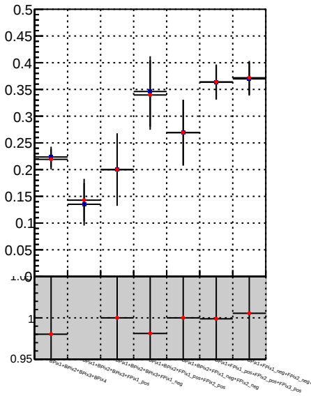
Fake rate vs. \bullet DQM TT mkFit-DQM_init_orig \bullet DQM TT mkFit-DQM_init_mod
