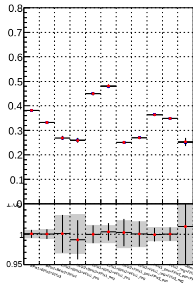
Fake rate vs. —●— DQM TT mkFit-DQM_init_orig —●— DQM TT mkFit-DQM_init_mod
