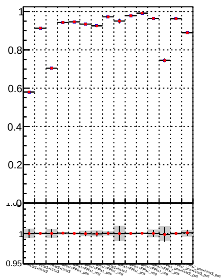
Fake rate vs. —●— DQM TT mkFit-DQM_init_orig —●— DQM TT mkFit-DQM_init_mod
