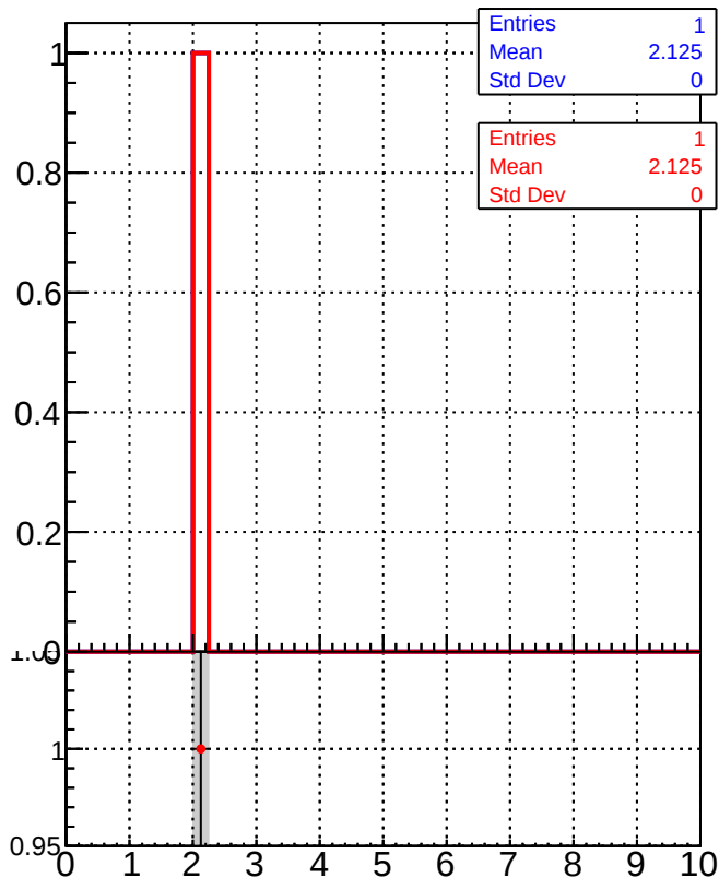
dE/dx estimator 1
