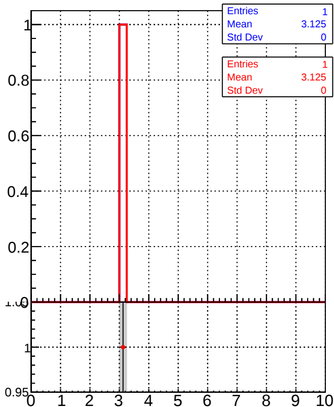
dE/dx estimator 2
