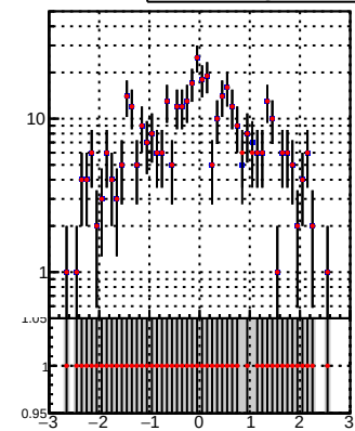
DQM TT mkFit-DQM_init_orig DQM TT mkFit-DQM_init_modi3
