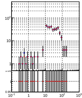
DQM TT mkFit-DQM_init_orig DQM TT mkFit-DQM_init_modi3
