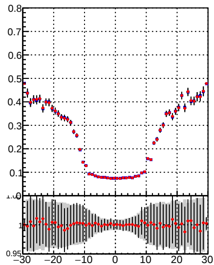
—•— DQM\_TT\_mkFit-DQM\_init\_orig —•— DQM\_TT\_mkFit-DQM\_init\_mod3
