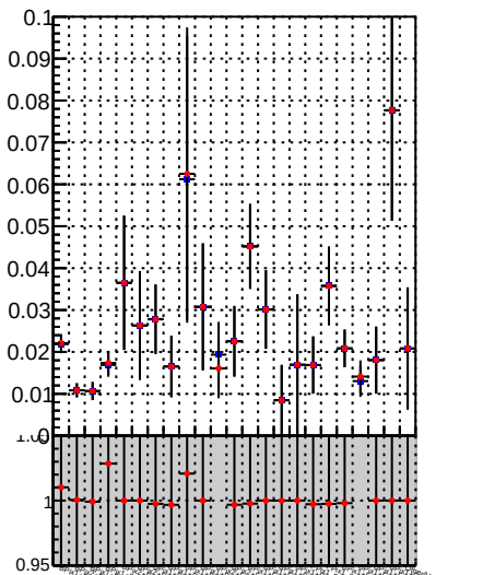
Fake rate vs. — DQM TT mkFit-DQM_init_orig — DQM TT mkFit-DQM_init_modi3
