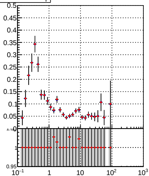
■ DQM\_TT\_mkFit-DQM\_init\_orig ● DQM\_TT\_mkFit-DQM\_init\_modi3
