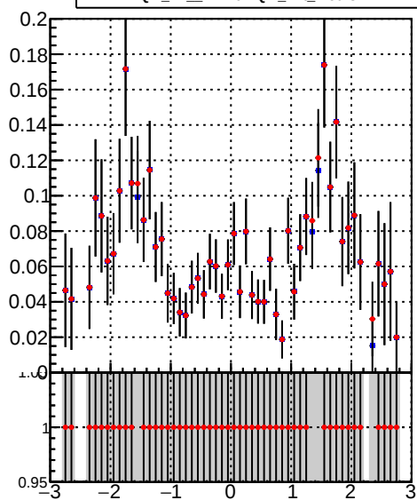
■ DQM\_TT\_mkFit-DQM\_init\_orig ● DQM\_TT\_mkFit-DQM\_init\_modi3
