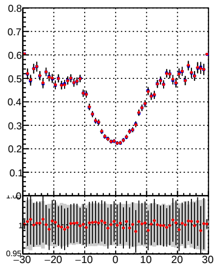
—●— DQM\_TT\_mkFit-DQM\_init\_orig —●— DQM\_TT\_mkFit-DQM\_init\_modi3
