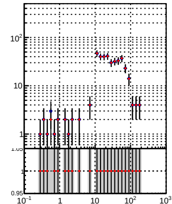
N of reco track vs \eta pT eta ● DQM TT mkFit-DQM_init_orig ● DQM TT mkFit-DQM_init_modi3
