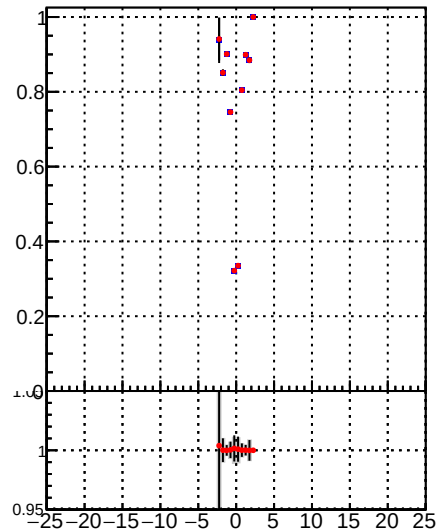
—•— DQM TT mkFit-DQM_init_orig —•— DQM TT mkFit-DQM_init_mod12
