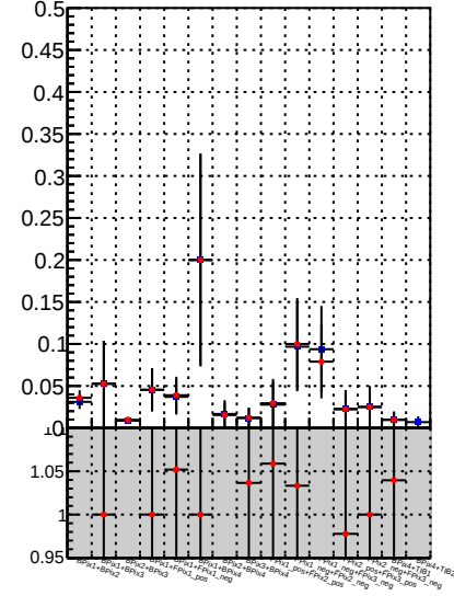
Fake rate vs. — DQM TT mkFit-DQM_init_orig — DQM TT mkFit-DQM_init_modi2
