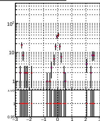
pT [GeV]
