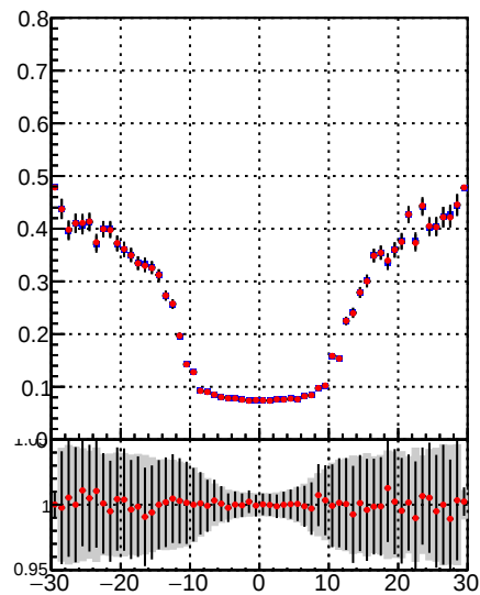
—•— DQM\_TT\_mkFit-DQM\_init\_orig —•— DQM\_TT\_mkFit-DQM\_init\_mod2
