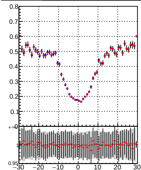
—•— DQM\_TT\_mkFit-DQM\_init\_orig —•— DQM\_TT\_mkFit-DQM\_init\_modi2
