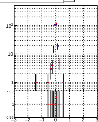
pT eta
