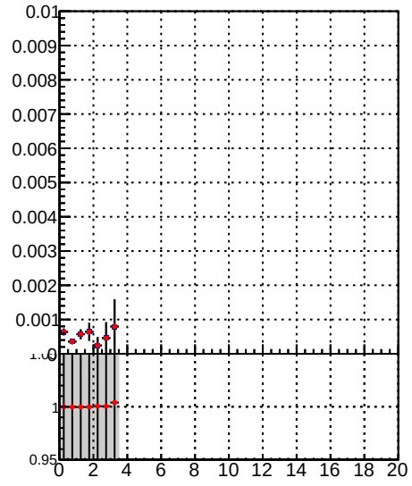
Fake rate vs. \chi^2 DQM TT mkFit-DQM_init_orig \chi^2 DQM TT mkFit-DQM_init_modi2
