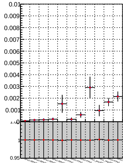
Fake rate vs. \chi^2 DQM TT mkFit-DQM_init_orig \chi^2 DQM TT mkFit-DQM_init_modi2
