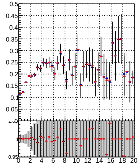
Fake rate vs. \chi^2 DQM TT mkFit-DQM_init_orig \chi^2 DQM TT mkFit-DQM_init_modi2
