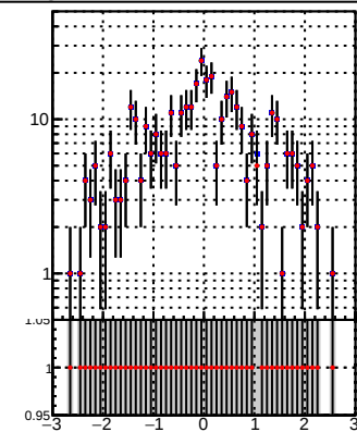
it-DQM_init_orig it-DQM_init_modi2
