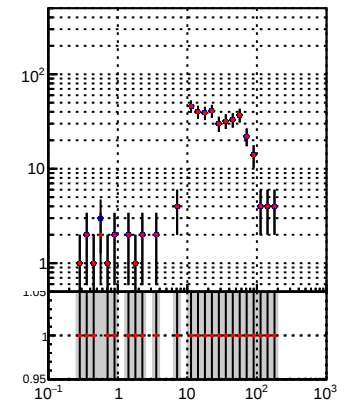
it-DQM_init_orig it-DQM_init_modi2
