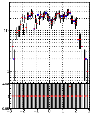
N of reco track vs \eta DQM TT mkFit-DQM_init_orig DQM TT mkFit-DQM_init_modi2
