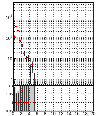
Legend: DQM TT mkFit-DQM_init_orig DQM TT mkFit-DQM_init_mod12
