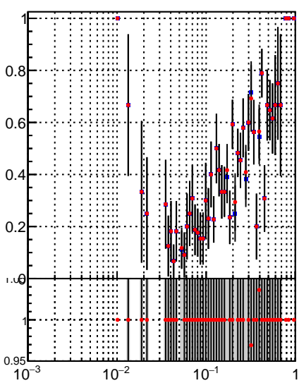
■ DQM_TT_mkFit-DQM_init_orig ■ DQM_TT_mkFit-DQM_init_modi2
