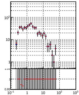
—•— DQM TT mkFit-DQM_init_orig —•— DQM TT mkFit-DQM_init_modi2
