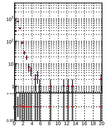
N of reco track vs. \chi^2 DQM TT mkFit-DQM_init_orig DQM TT mkFit-DQM_init_mod12
