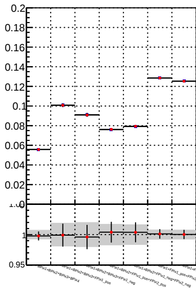
Fake rate vs. —●— DQM TT mkFit-DQM_init_orig —●— DQM TT mkFit-DQM_init_modi2
