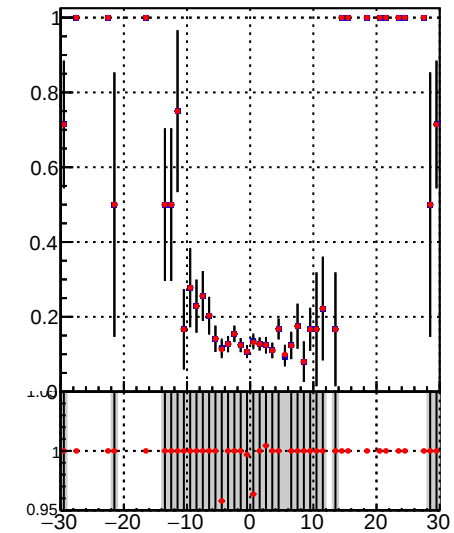
—●— DQM\_TT\_mkFit-DQM\_init\_orig —●— DQM\_TT\_mkFit-DQM\_init\_modi2
