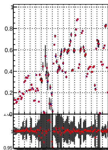
Fake rate vs. —●— DQM TT mkFit-DQM_init_orig —●— DQM TT mkFit-DQM_init_modi
