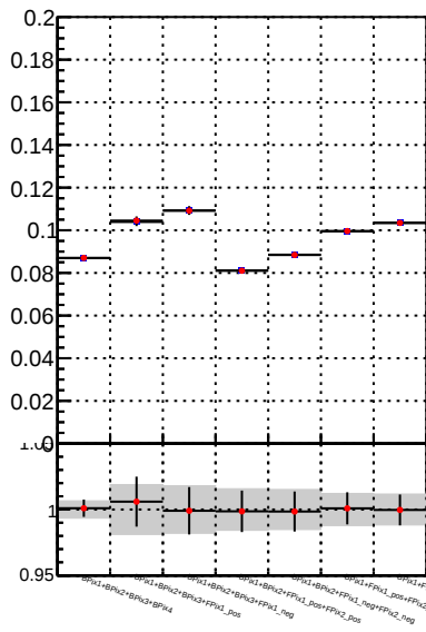
Fake rate vs. DQM TT mkFit-DQM_init_orig DQM TT mkFit-DQM_init_modi
