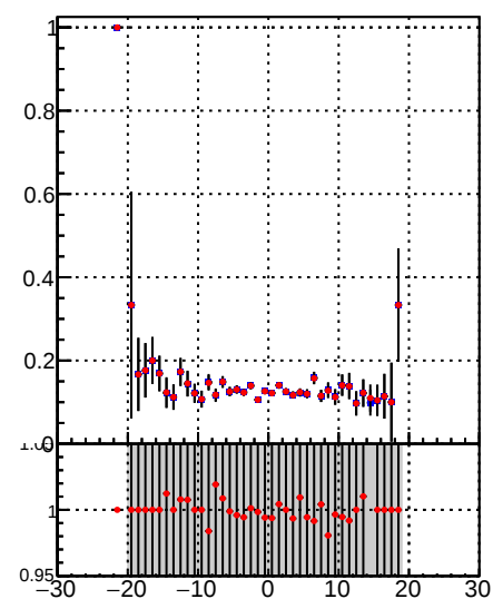
Fake rate vs d —•— DQM TT mkFit-DQM_init_orig —•— DQM TT mkFit-DQM_init_modi
