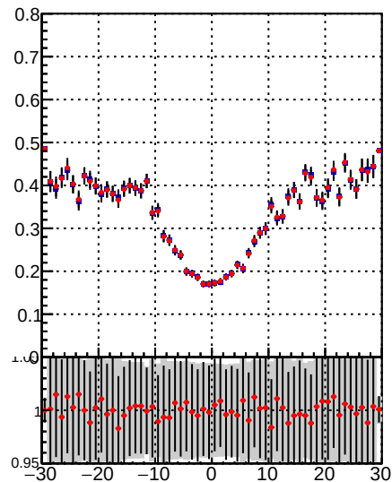
—●— DQM\_TT\_mkFit-DQM\_init\_orig —●— DQM\_TT\_mkFit-DQM\_init\_modi
