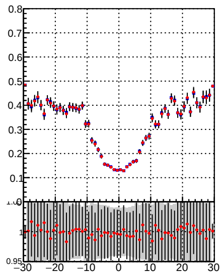
—•— DQM TT mkFit-DQM_init_orig —•— DQM TT mkFit-DQM_init_modi
