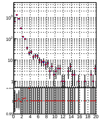
Legend: DQM TT mkFit-DQM_init_orig DQM TT mkFit-DQM_init_modi
