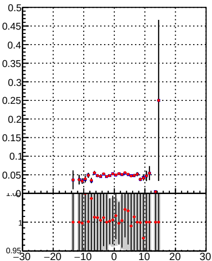
Fake rate vs \Delta y —•— DQM TT mkFit-DQM_init_orig —•— DQM TT mkFit-DQM_init_modi
