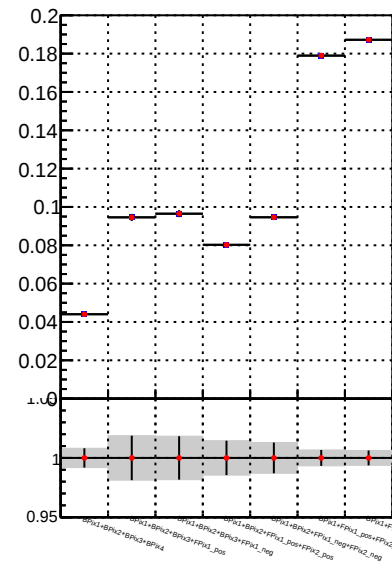
Fake rate vs. \chi^2 DQM TT mkFit-DQM_init_orig \chi^2 DQM TT mkFit-DQM_init_modi
