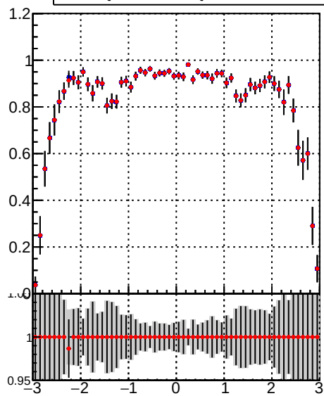
■ DQM_TT_mkFit-DQM_init_orig ■ DQM_TT_mkFit-DQM_init_modi
