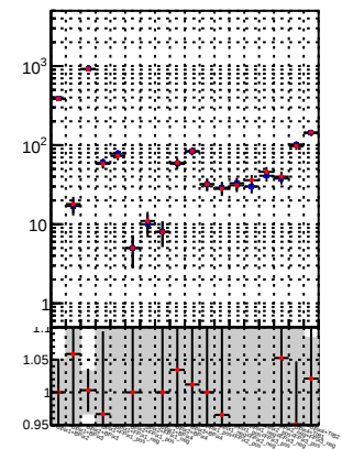
N of reco track vs. \chi^2 DQM TT mkFit-DQM_init_orig DQM TT mkFit-DQM_init_modi
