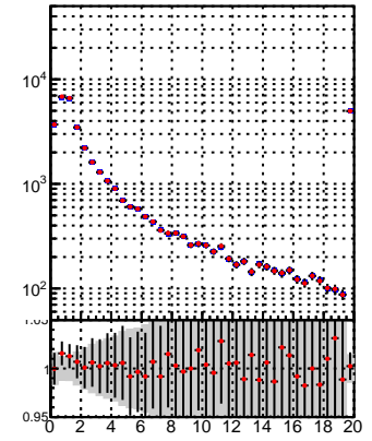
N of reco track vs. \chi^2 —●— DQM TT mkFit-DQM_init_orig —●— DQM TT mkFit-DQM_init_mod
