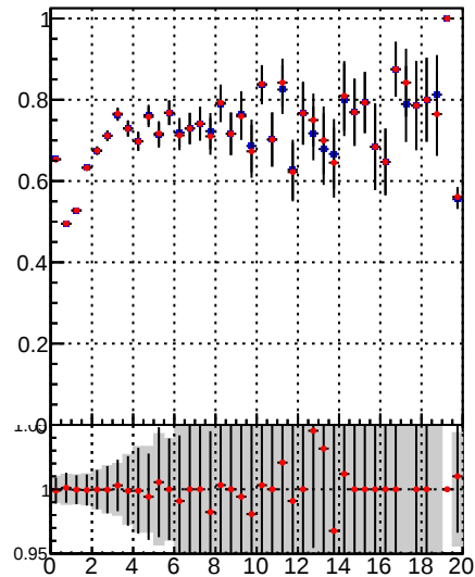
Fake rate vs. \chi^2 DQM TT mkFit-DQM_init_orig \chi^2 DQM TT mkFit-DQM_init_modi
