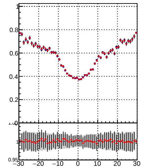
—●— DQM TT mkFit-DQM_orig2 —●— DQM TT mkFit-DQM_mod2
