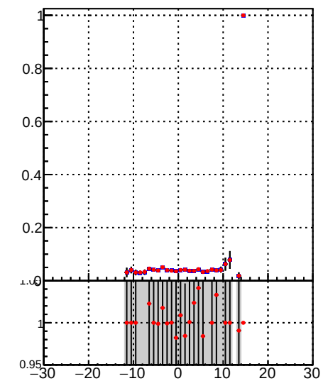
Fake rate vs d DQM TT mkFit-DQM_orig2 DQM TT mkFit-DQM_mod2
