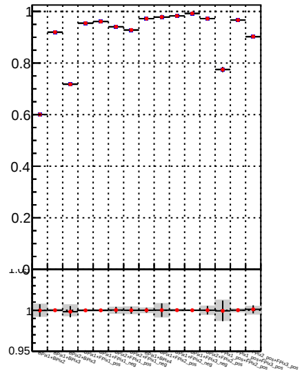
Fake rate vs. —●— DQM TT mkFit-DQM_orig2 —●— DQM TT mkFit-DQM_mod2
