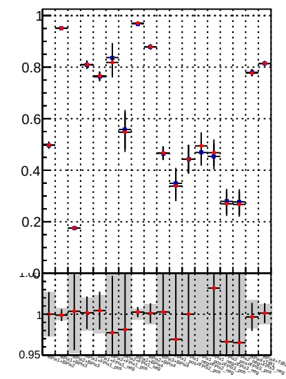
Fake rate vs. \bullet DQM TT mkFit-DQM_orig2 \bullet DQM TT mkFit-DQM_mod2
