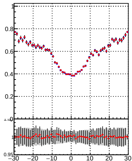
—●— DQM TT mkFit-DQM_orig2 —●— DQM TT mkFit-DQM_mod2
