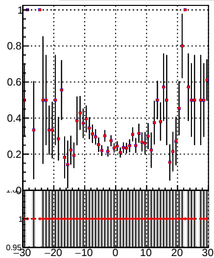
█ DQM_TT_mkFit-DQM_orig █ DQM_TT_mkFit-DQM_mod
