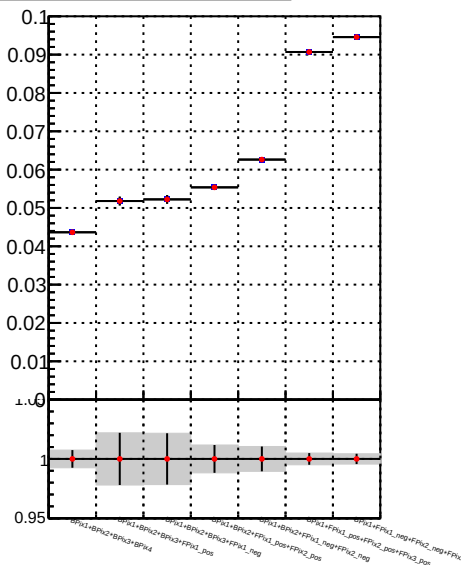
Fake rate vs. —•— DQM TT mkFit-DQM_orig —•— DQM TT mkFit-DQM_mod
