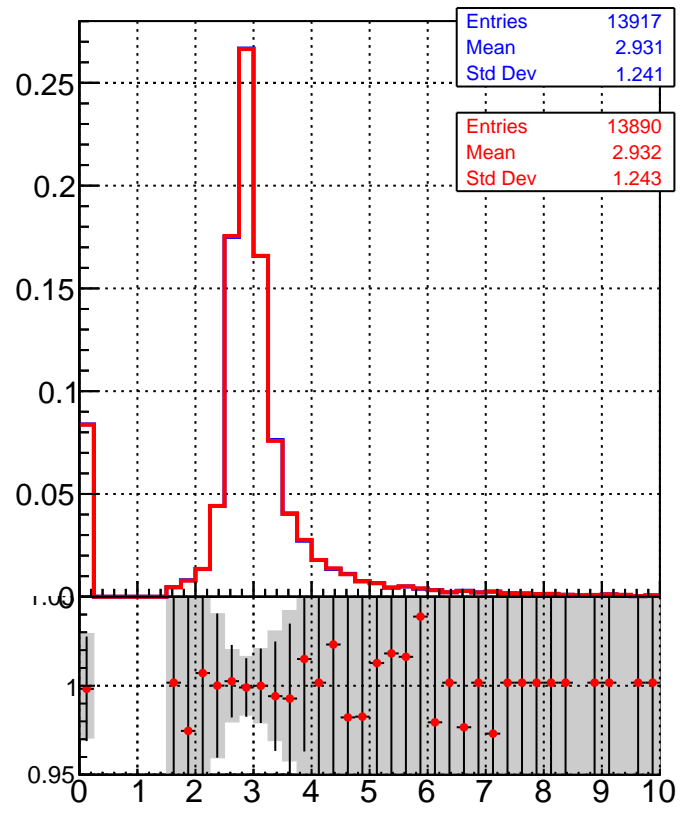
dE/dx estimator 2
