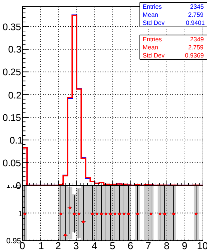
dE/dx estimator 2
