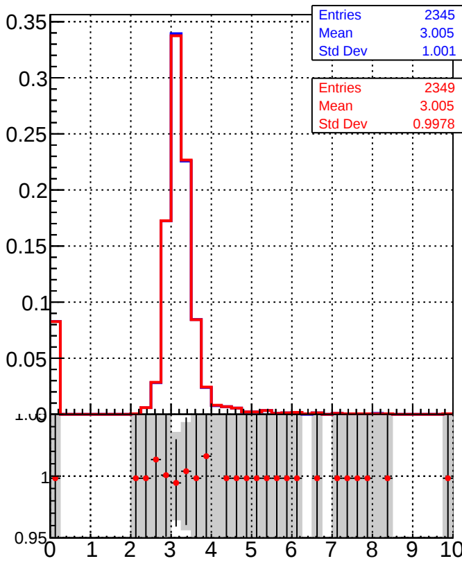
dE/dx estimator 1
